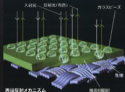
再帰反射メカニズム
